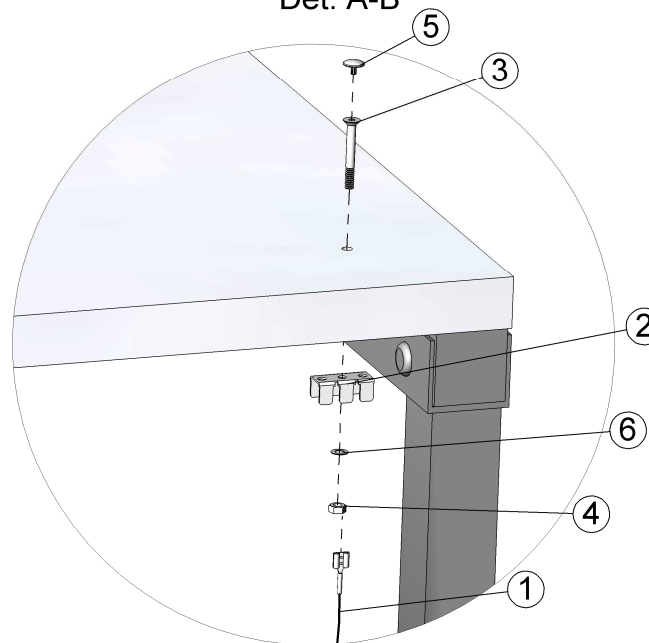
Det. A-B
